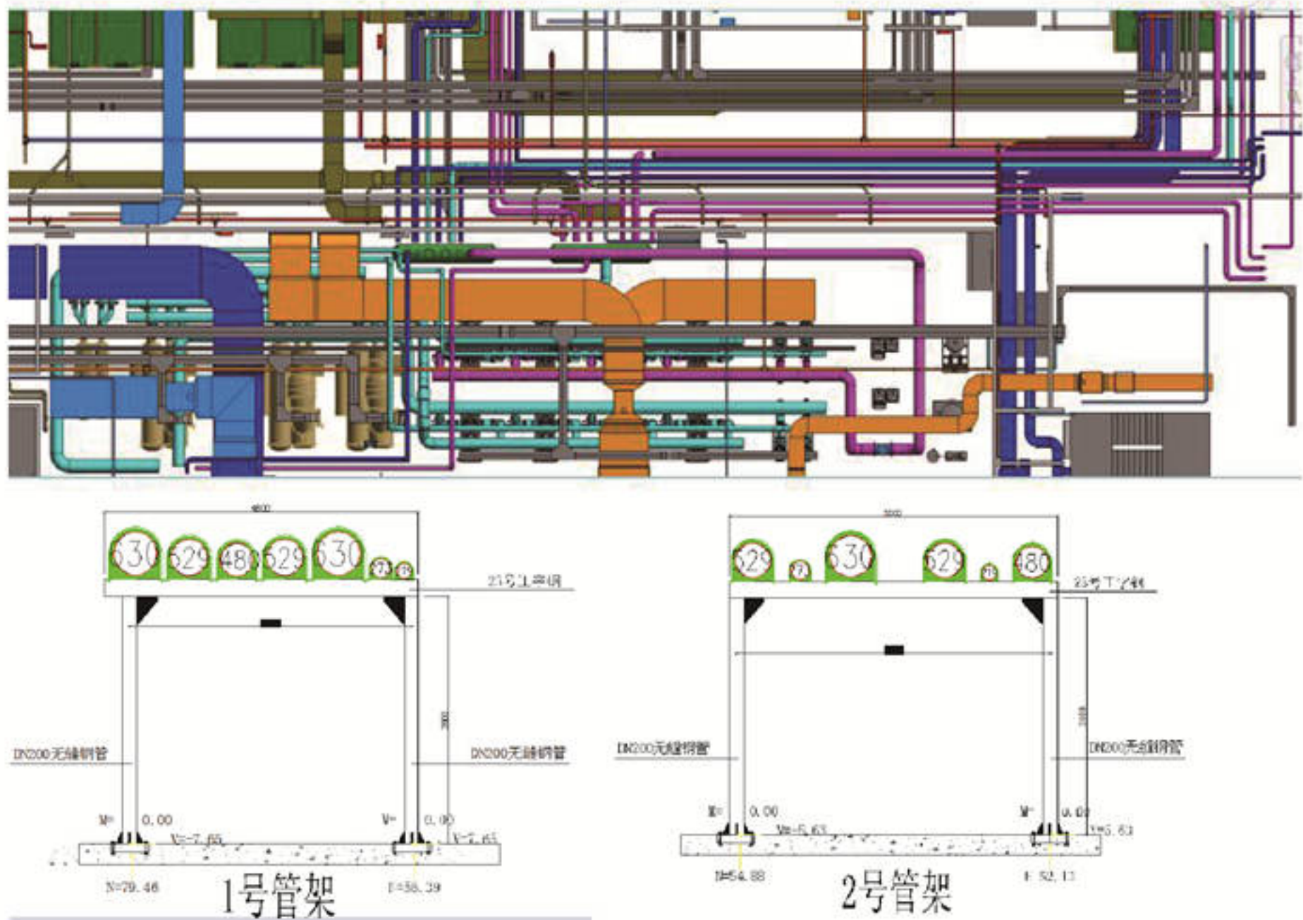
图4平面图，三维图，剖面图，支吊架图
