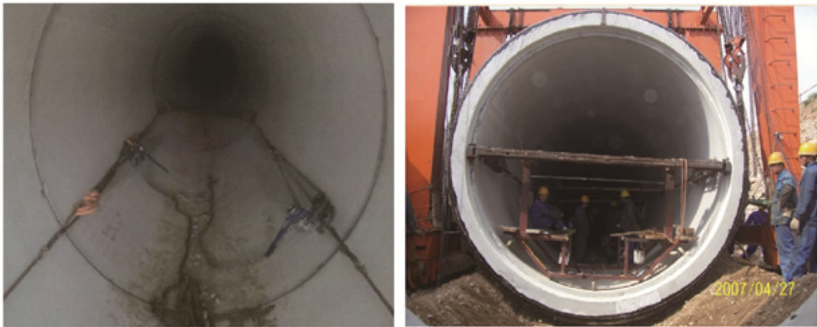
手拉葫芦对接内拉法实例
