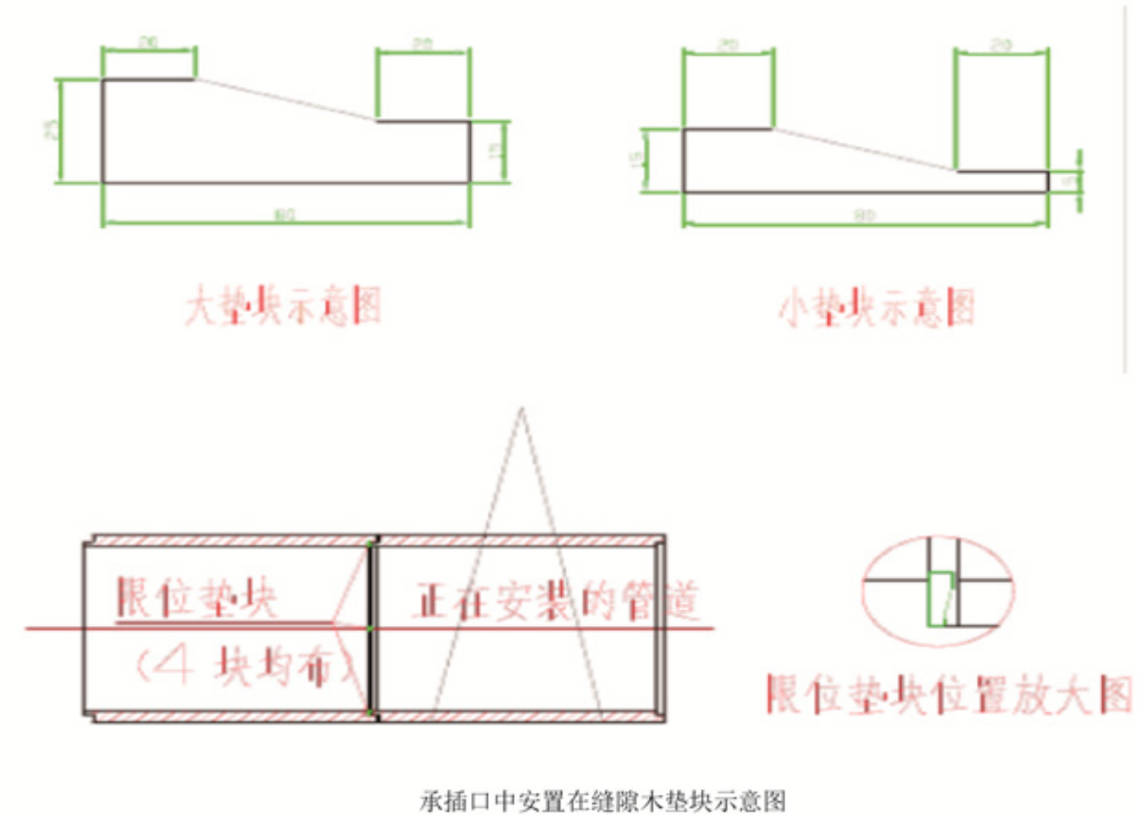
承插口中安置在缝隙木垫块示意图
